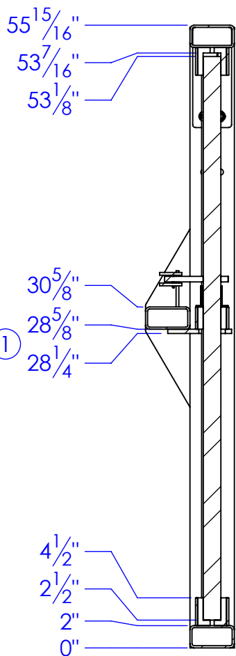
SECTION B-B SCALE 1 : 12
